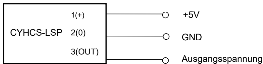
Bild. 4 Verbindung von CYHCS-LSP
